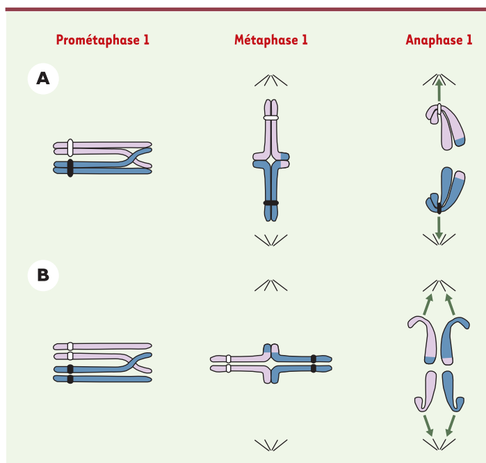
Figure 4. Configuration d'une paire de chromosomes acrocentriques présentant un échange chiasmatique en prométaphase I, métaphase I et anaphase I. A. En présence de cohésine, l'orientation stable du bivalent sur le fuseau assure une séparation parfaite des deux chromosomes. B. En l'absence de cohésion, le bivalent adopte une configuration linéaire, plus stable mais favorisant la ségrégation indépendante et prématurée de chaque chromatide (d'après [20]).
