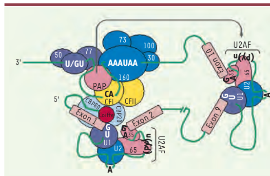
Figure 4. Interaction entre les processus de maturation de l'ARNm.
