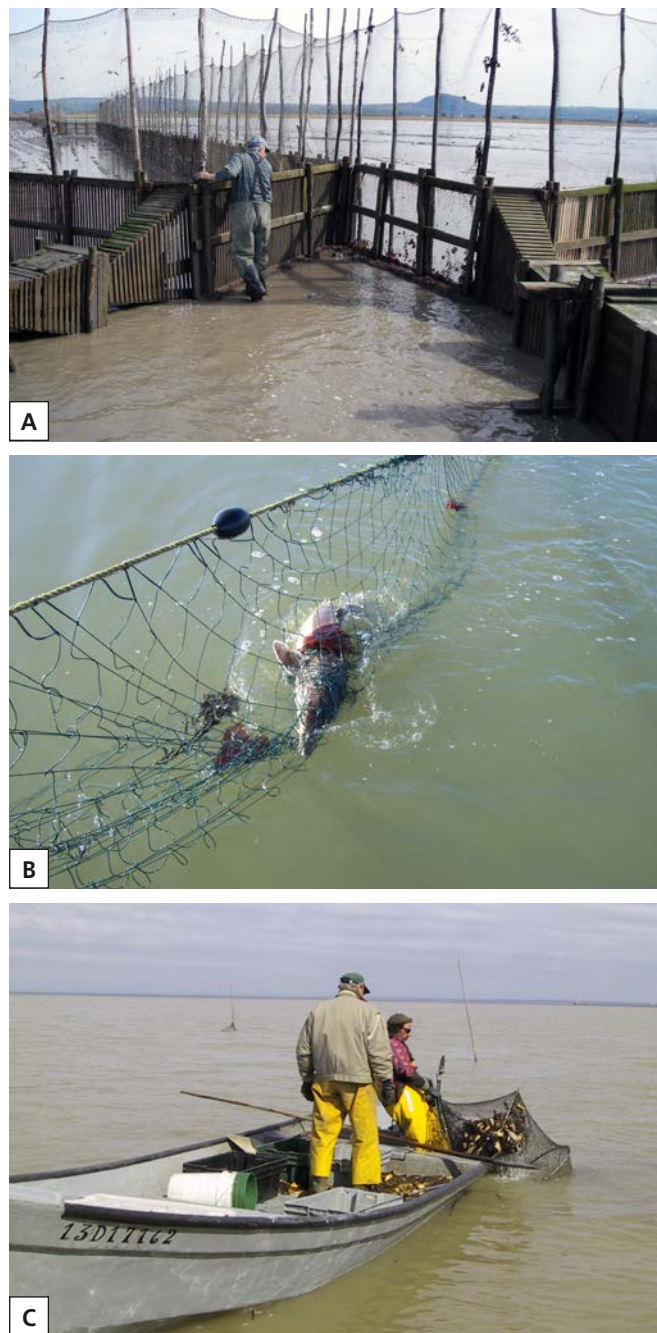
Figure 2. Illustrations des types d'engins de pêche utilisés par les pêcheurs commerciaux participant au Réseau de détection des espèces aquatiques exotiques envahissantes dans le fleuve Saint-Laurent: A) trappes fixes à anguille; B) filets maillants; C) verveux.
