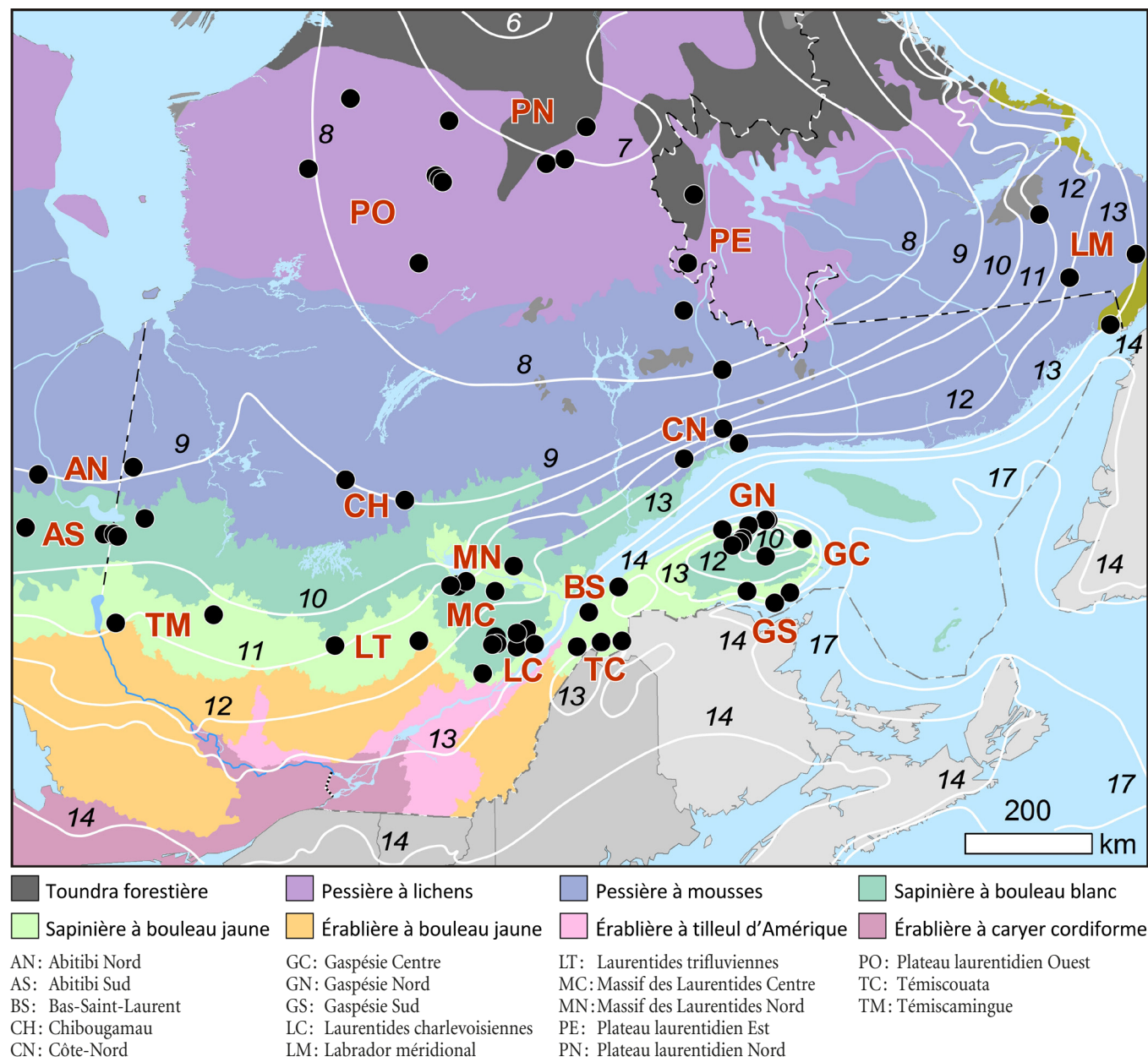
Figure 1. Répartition des lacs (points noirs) dont les sédiments ont livré des diagrammes polliniques et identification des 18 secteurs de la figure 3 dans les divers domaines bioclimatiques de la forêt boréale du Québec et du Labrador selon Saucier et collab. (2009) et selon Baldwin et collab. (2018) pour le Labrador et l'Ontario. Les lignes blanches isochrones de la dernière déglaciation (Dyke et collab., 2003; mis à jour) sont tracées à tous les 1000 ans avant l'Actuel (soit l'année 1950 de notre ère, par convention), sauf pour 17 ka AA dans le golfe du Saint-Laurent. Le nombre en caractères italiques au-dessus de chaque isochrone en indique l'âge.
