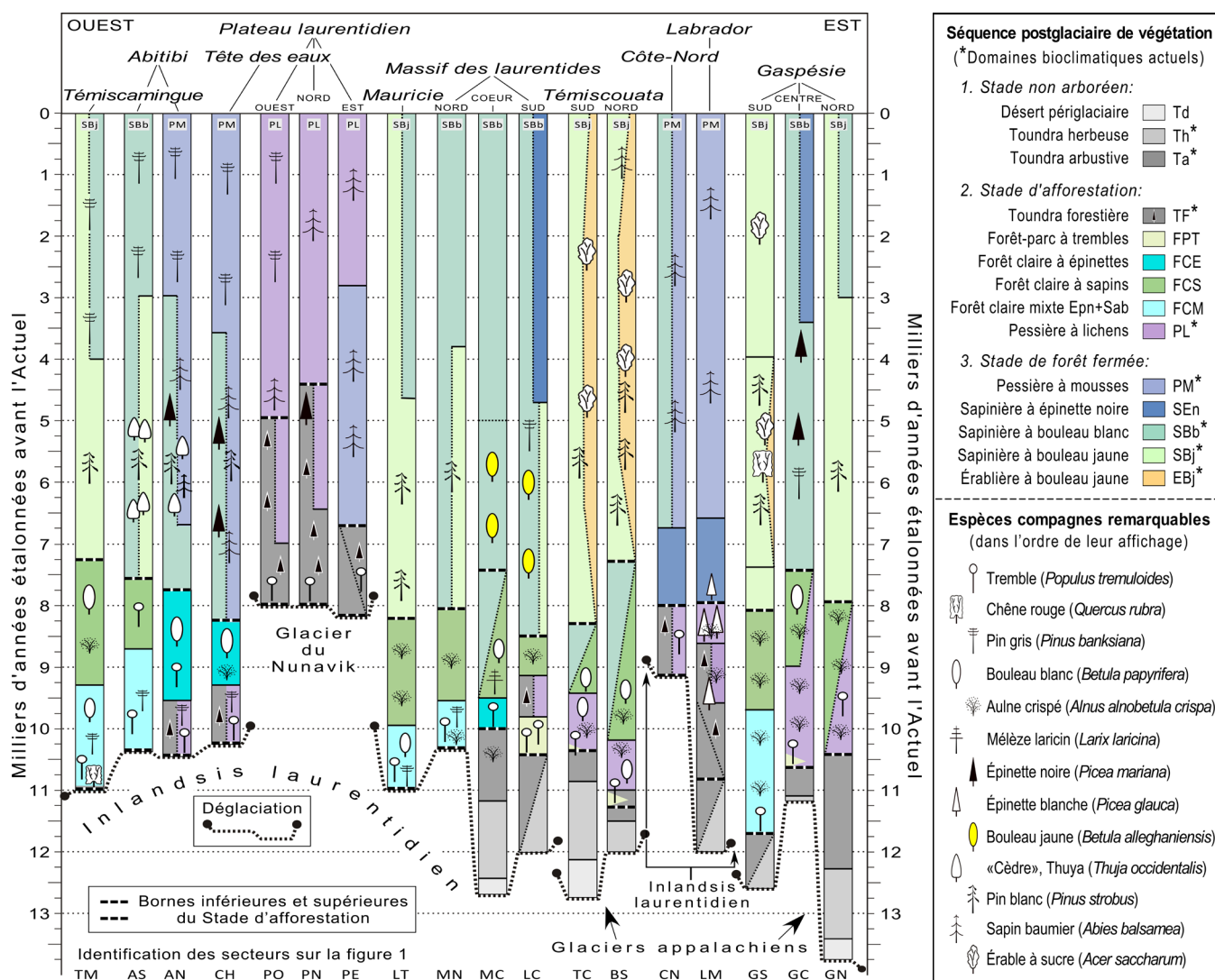
Figure 3. Séquences postglaciaires de la végétation des 18 secteurs (ou régions) de la forêt boréale du Québec et du sud du Labrador qui apparaissent sur la figure 1. Les secteurs sont identifiés au bas de la figure. Ils sont ordonnés d'ouest en est, et le territoire dont ils proviennent est mentionné au haut de la figure. L'espace plus large entre les séquences distingue les régions. Le sigle du domaine de végétation actuel figure au sommet des séquences. L'échelle de temps est reproduite des deux côtés en milliers d'années avant l'Actuel (soit l'année 1950 de notre ère, par convention). La légende graphique accompagnant la figure livre la séquence étalon des formations végétales (toundras) et des domaines de végétation qui apparaissent sur les colonnes. Elle montre aussi des pictogrammes positionnés à l'époque où certaines essences atteignent une abondance particulièrement élevée dans les paysages végétaux reconstitués.
