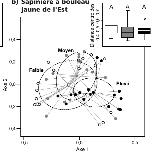
Figure 3. Dispersion multivariée (diversité bêta) entre les parcelles avec un niveau de couvert forestier faible (0 à 3 %), moyen (15 à 40 %) et élevé (> 60 %) dans les tourbières ombrotrophes uniformes a) des domaines bioclimatiques des érablières et b) du sous-domaine de la sapinière à bouleau jaune de l'Est au Québec. Les résultats sont présentés à l'aide des 2 premiers axes d'une analyse en coordonnées principales. Les ovales pointillés représentent les ellipses des écarts-types. Les diagrammes à moustaches (en mortaise) représentent la dispersion des distances des placettes par rapport au centroïde pour chaque groupe. Les lignes supérieure, centrale et inférieure de la boîte à moustaches correspondent respectivement au 75 e , au 50 e et au 25 e percentile. Les extrémités des moustaches sont calculées en utilisant 1,5 fois l'espace interquartile (la distance entre le 1 er et le 3 e quartile). Les valeurs à l'extérieur des moustaches sont représentées par des points, et correspondent généralement à des valeurs extrêmes. Les groupes dont la diversité bêta est significativement différente sont indiqués par les lettres majuscules A et B.
