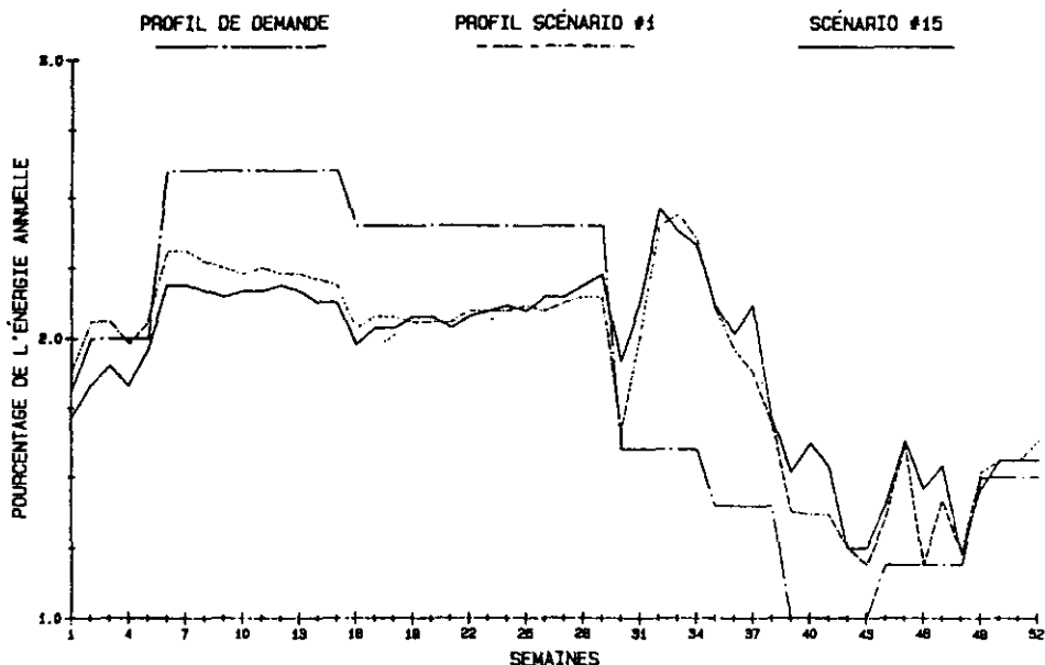
Figure 3.- Comparaison des profils de production pour le scénario #1 sans contrainte et pour le scénario #15 avec contrainte au niveau de fiabilité acceptable.
