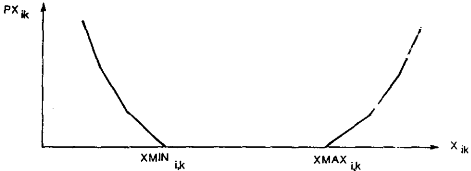
Figure 1.- Fonctions de pénalités.
