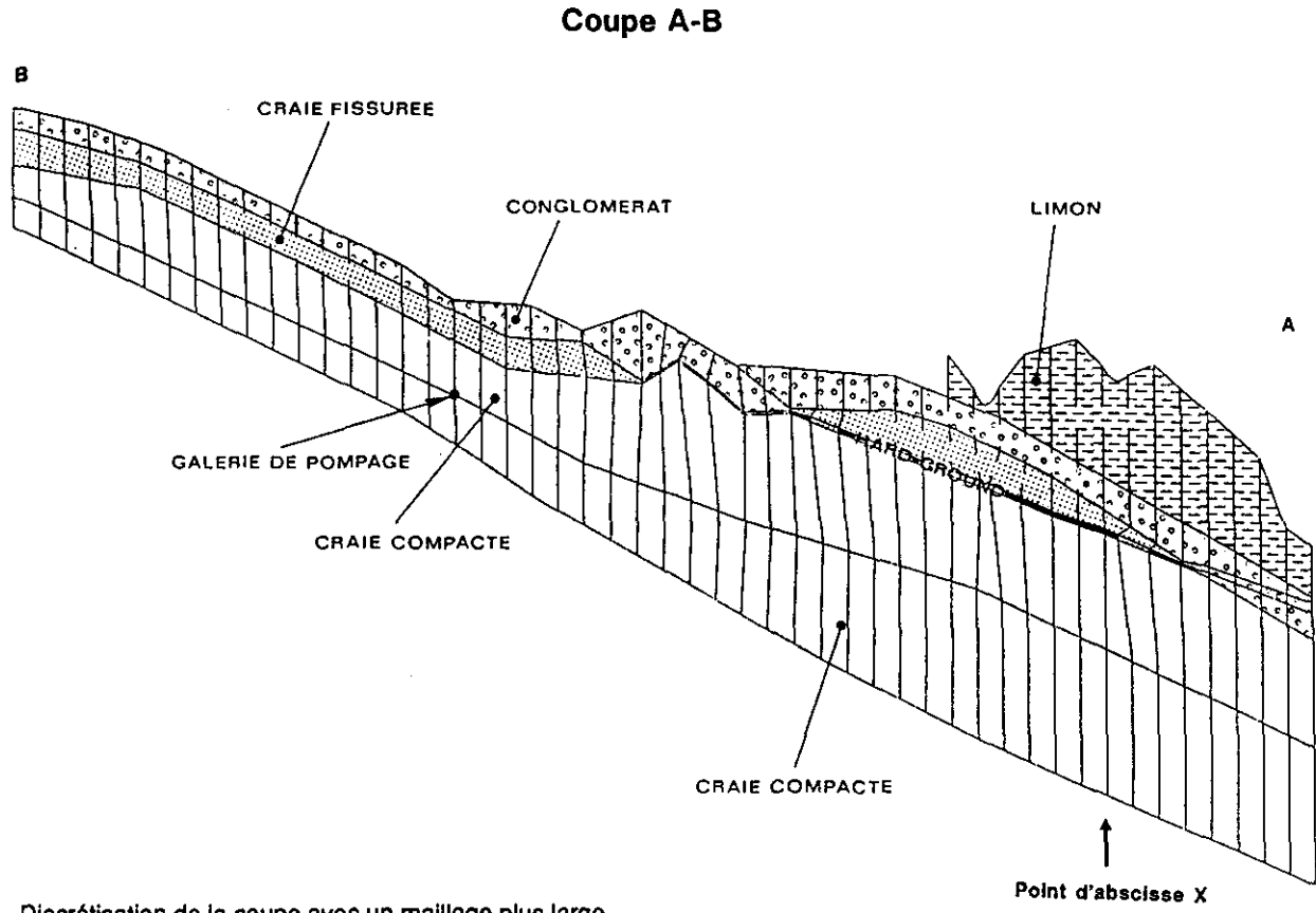
Figure 8 Discretisation de la coupe avec un maillage plus large. Wide meshing discretization of the vertical cross-section.
