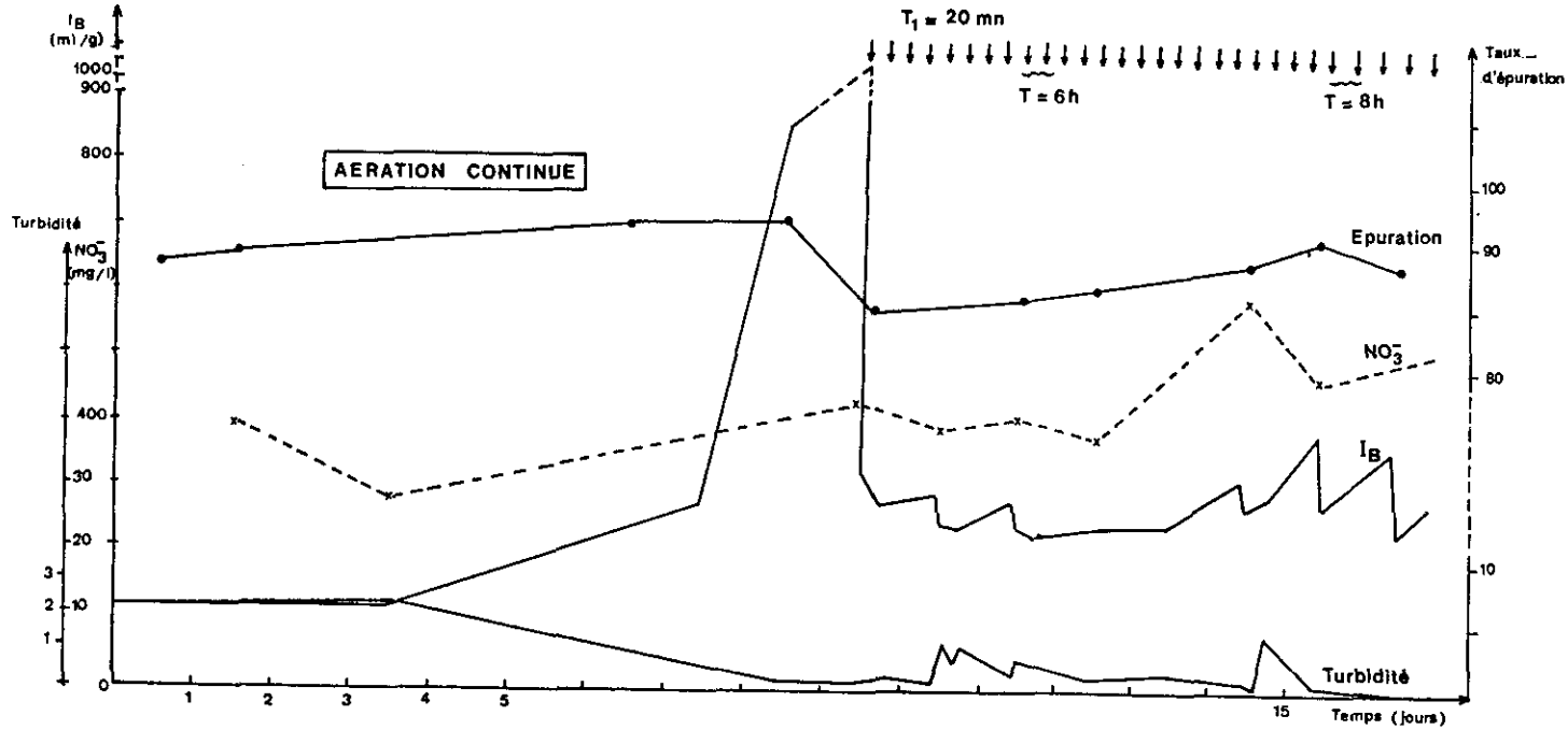
Figure 5 Evolution de I_B , DCO, NO_3^- et de la turbidité en fonction du temps pour Re = 0,71 \cdot 10^5 , T_1 = 20\text{ mn} , t = 6\text{ h} , 8\text{ h} (aération continue).
