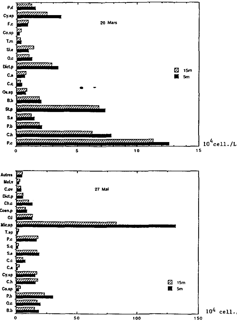
Figure 3 Densités des espèces phytoplanctoniques à 5 et à 15 m le 20 mars et le 27 mai 1992.
