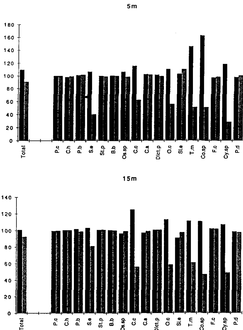
Figure 4 Évolution de la densité du peuplement phytoplanctonique global et des principales composantes (en % de N_{t_0} ) en absence (noir) et en présence (gris) de zooplancton après 8 heures d'incubation (20 mars 1992).
