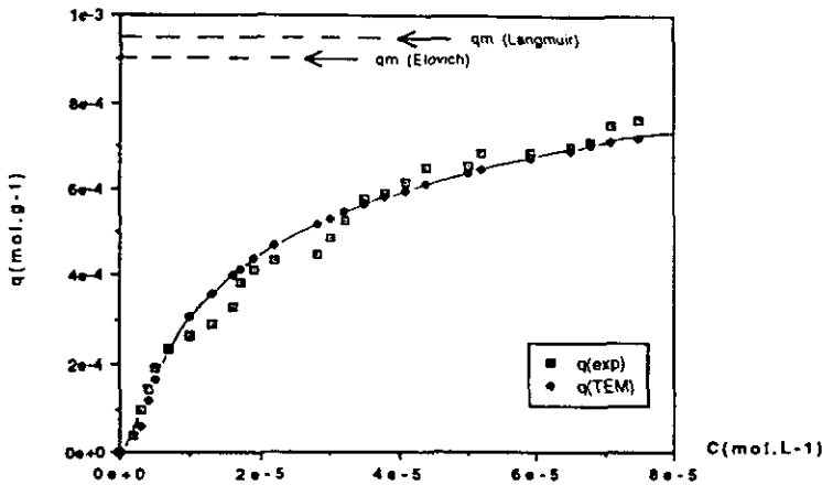
Figure 7 Comparaison des capacités d'adsorption expérimentales et calculées par l'équation de TEMKIN pour la phénylalanine. Comparison of experimental and calculated adsorption capacities for the different equations, for phenylalanine.
