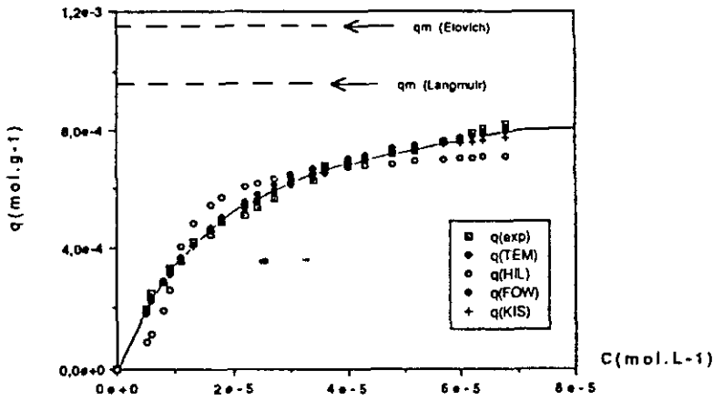
Figure 6 Comparaison des capacités d'adsorption expérimentale et calculée par les différentes équations pour la tyrosine. Comparison of experimental and calculated adsorption capacities, for the different equations, for tyrosine.
