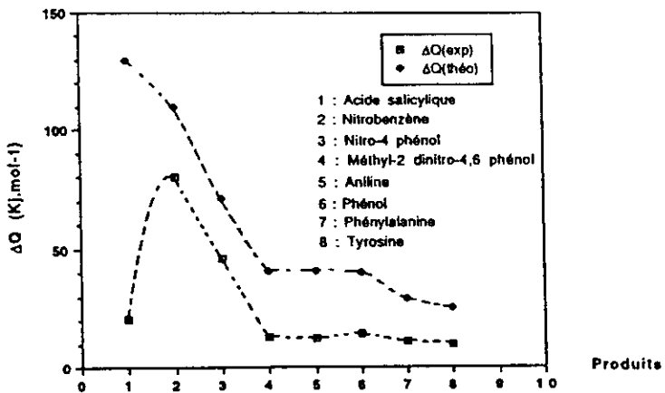
Figure 9 Evolution de la variation d'énergie d'adsorption ΔQ de TEMKIN en fonction de la structure du produit.
