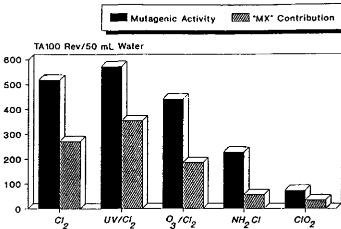
Figure 1 Activité mutagène (Rev./50 mL) et contribution du MX à la mutagenicité calculée dans l'eau du lac Savojarvi (COD: 20 mg/L) après traitement avec divers désinfectants. Doses initiales des désinfectants: Cl 2 : 20 mg/L; UV/Cl 2 : 12 min/20 mg/L; O 3 /Cl 2 : 30 mg/L/20 mg/L; NH 2 Cl: 10 mg/L; ClO 2 : 20 mg/L.
