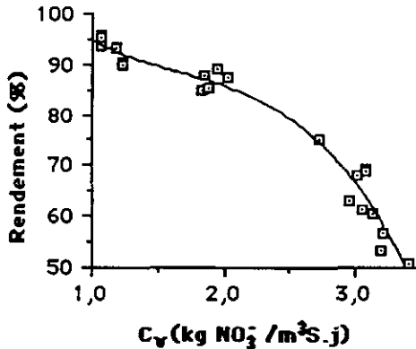
Figure 4 Influence de la charge volumique sur le rendement de dénitrification à 20 \pm 1 °C.
