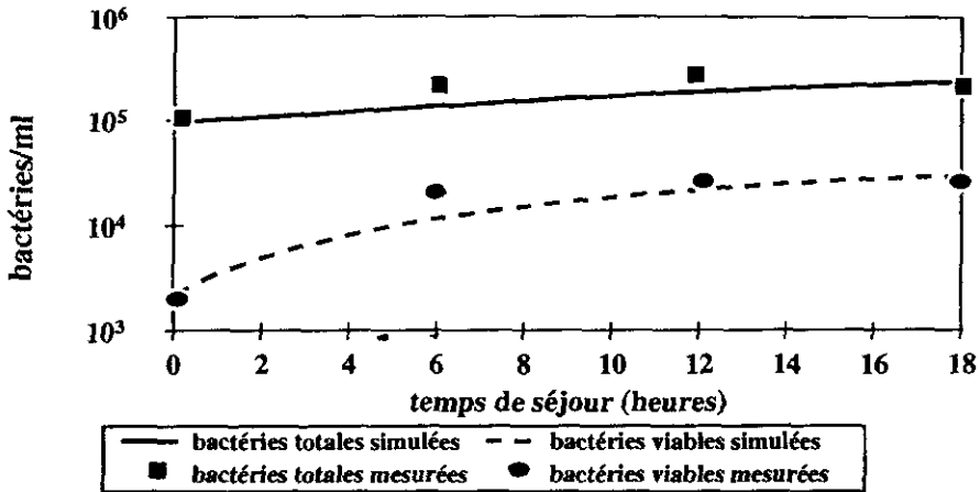
Figure 5 Validation du modèle sur pilote – comparaison entre les valeurs mesurées et simulées pour la flore libre viable et totale ( t^{\circ} : 20 °C ; CODB : 0,45 ppm). Comparison between measurements and simulation for viable and total free bacteria ( T : 20°C; BDOC: 0.45 ppm).
