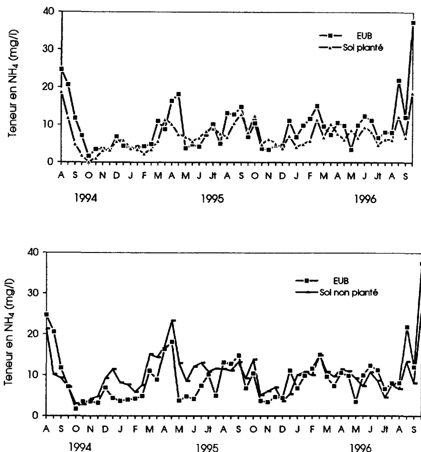
Figure 8 Évolution temporelle de la teneur en ions ammoniums à l'entrée et à la sortie du lit planté et du lit non planté.
