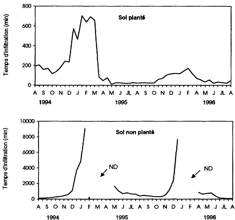
Figure 2 Évolution temporelle du temps d'infiltration de la lame d'eau (25 L) dans le lit planté et le sol non planté.
