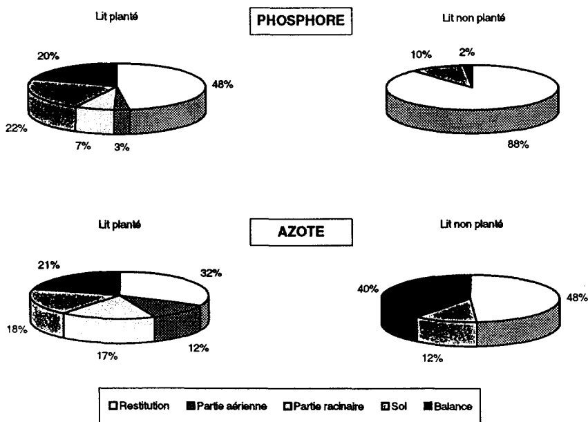
Figure 16 Bilan de l'azote et du phosphore au niveau des deux systèmes planté et non planté.
