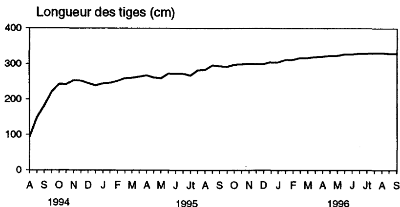
Figure 15 Évolution temporelle de la longueur des tiges du roseau. Temporal changes in the lenght of the reeds.
