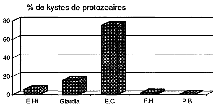
Figure 13 Pourcentage des différents types de kystes de protozoaires dans les eaux usées brutes. E.Hi.: Entamoeba histolitica , Giardia : Giardia sp., E.C.: Entamoeba coli , E.C.: Entamoeba hartmani , P.B.: Pseudolimax butshlin .
