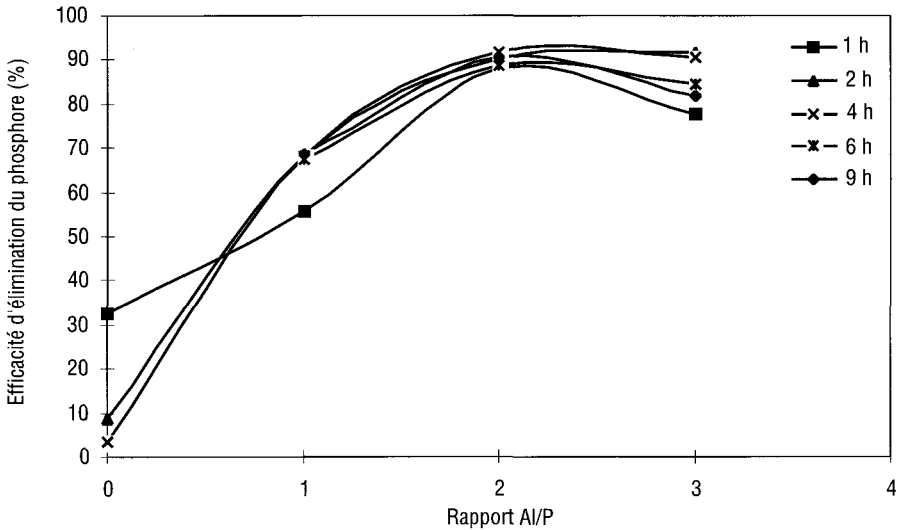
Figure 2 Efficacité d'élimination du phosphore en fonction du rapport massique Al/P ( V_f = 5 \text{ m/h} ; T_f = 10 \text{ min} ; \text{pH} = 6,5 ; C_p = 2 \text{ mg/l} ; G = 50 \text{ s}^{-1} ). Efficiency of phosphorus removal against Al/P mass ratios.
