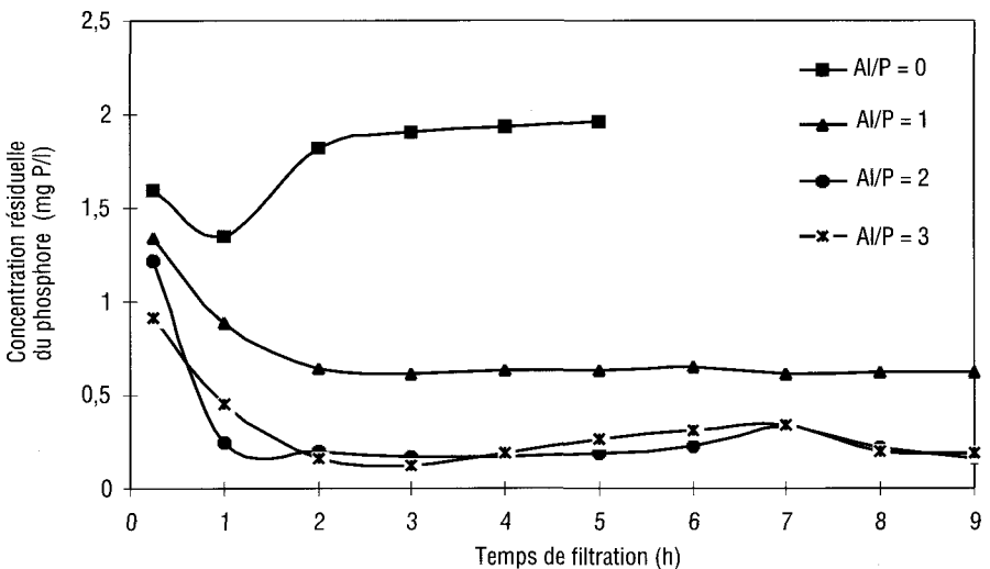
Figure 3 Variation de la concentration résiduelle du phosphore en fonction du temps de filtration et du rapport massique Al/P ( V_f = 5 \text{ m/h} ; T_f = 10 \text{ min} ; \text{pH} = 6,5 ; C_p = 2 \text{ mg/l} ; G = 50 \text{ s}^{-1} ). Variation of phosphorus residual concentration against filtration time and Al/P mass ratios.
