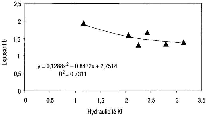
Figure 7 Variation de l'exposant (b) en fonction de l'Hydraulicité Ki (années humides).
