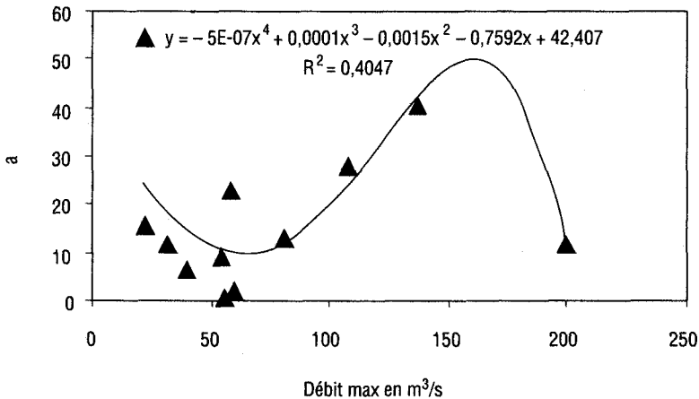
Figure 23 Variation du paramètre (a) en fonction du débit max. de la crue.
