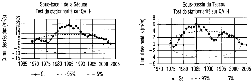
Figure 18 Rupture de stationnarité des modules d'hiver des sous-bassins de la Séoune et du Tescou. Stationnarity break in mean annual winter discharge time series for the Séoune and Tescou sub-basins.
