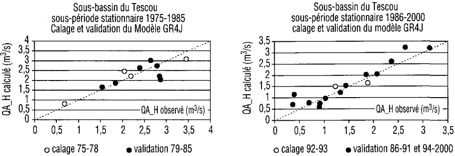
Figure 22 Calage et validation de GR4J sur les sous-périodes stationnaires des QA_H du Tescou. Calibration and validation of the GR4J model on QA_H stationary sub-periods for the Tescou sub-basin.
