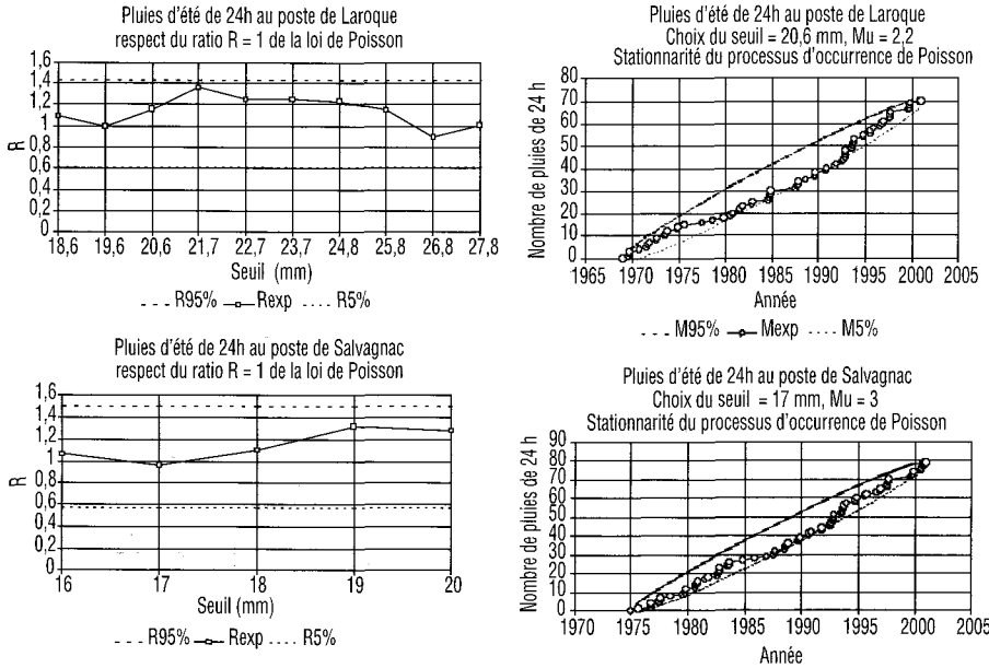
Figure 9 Stationnarité des pluies maximales d'été. Stationnarity of maximum summer rainfalls.
