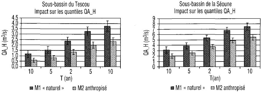
Figure 23 Quantiles et I.C. à 90 % des modules d'hiver des sous-bassins « naturels » et anthropisés.
