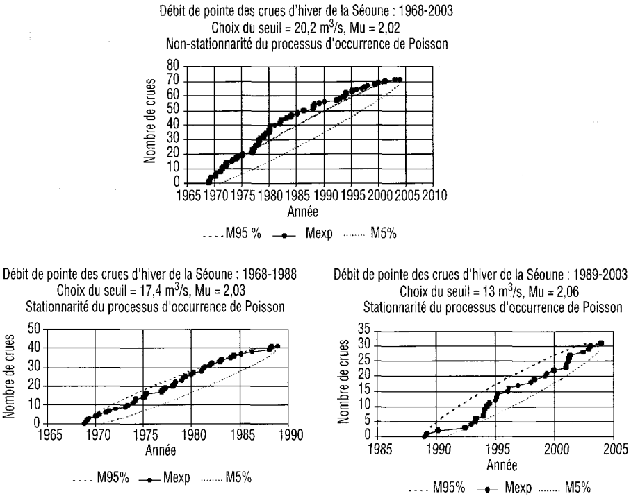
Figure 5 Séoune – Chronique des débits de pointe d'hiver non stationnaire, identification des 2 sous-périodes stationnaires.
