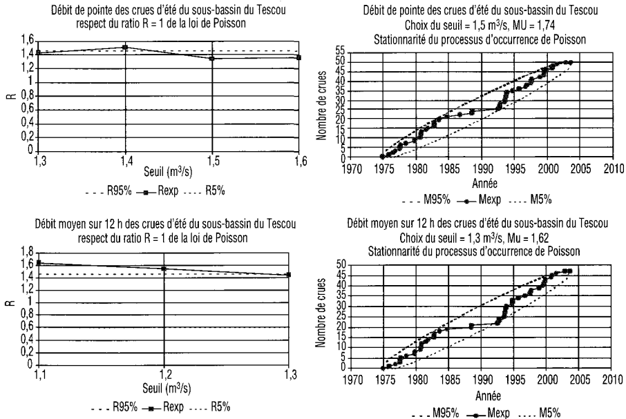
Figure 8 Stationnarité des chroniques de crue d'été du sous-bassin du Tescou.
