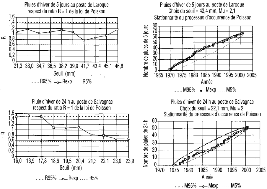
Figure 10 Stationnarité des pluies maximales d'hiver. Stationnarity of maximum winter rainfalls.
