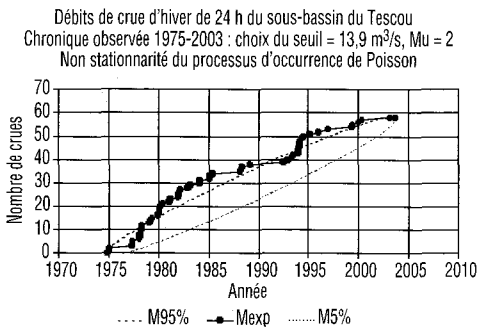
Figure 11 Non-stationnarité et stationnarité des crues de 24 h des chroniques respectives Q(t) et E_i (ex. : E_1 ).
