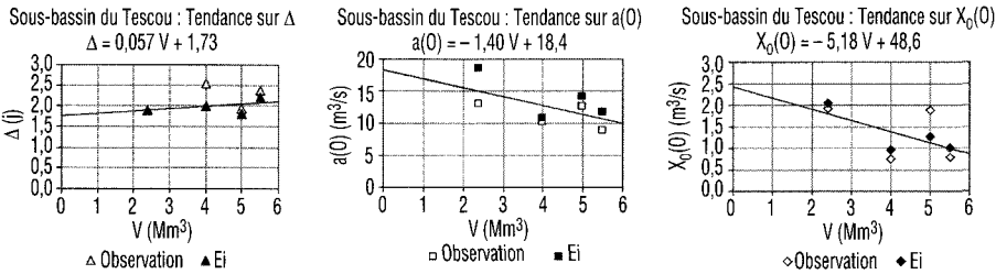
Figure 13 Tendance sur les paramètres des modèles QdF des crues d’hiver du Tescou. Tendency in QdF model parameters for winter floods in the Tescou sub-basin.
