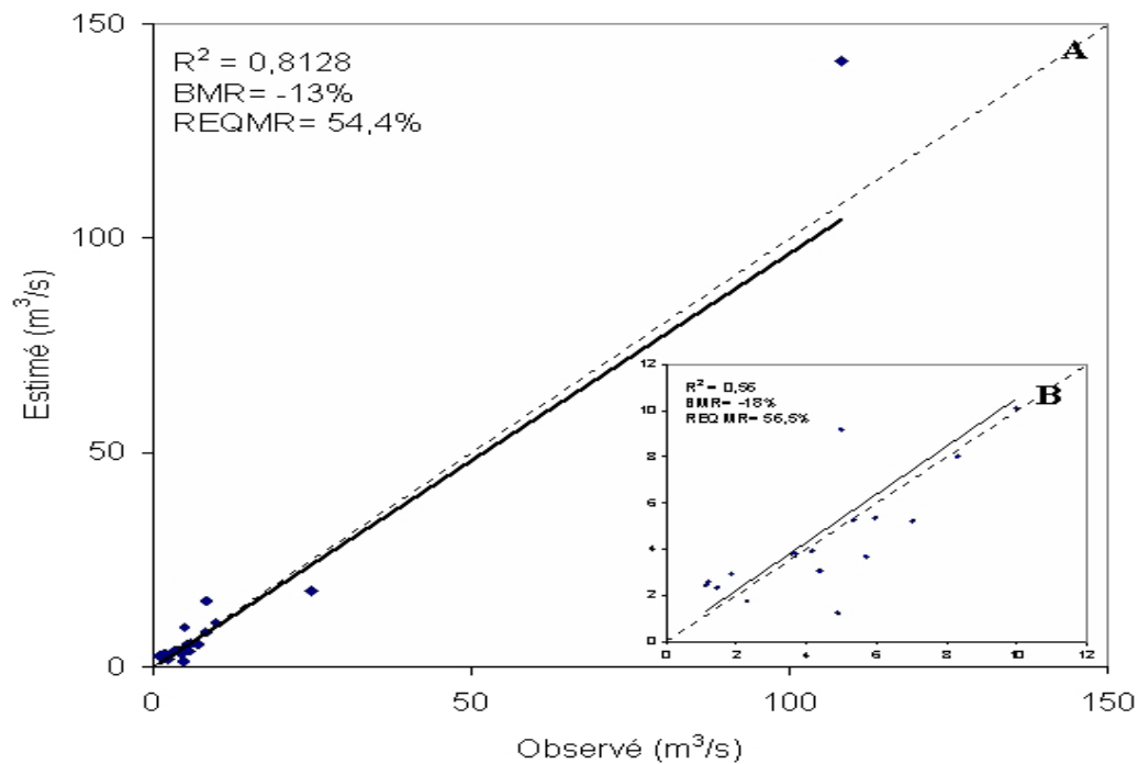
Figure 9 : Validation croisée du débit moyen interannuel estimé à l'aide du krigeage canonique : A) toutes les stations de jaugeage, B) excluant les trois plus grands bassins versants.
