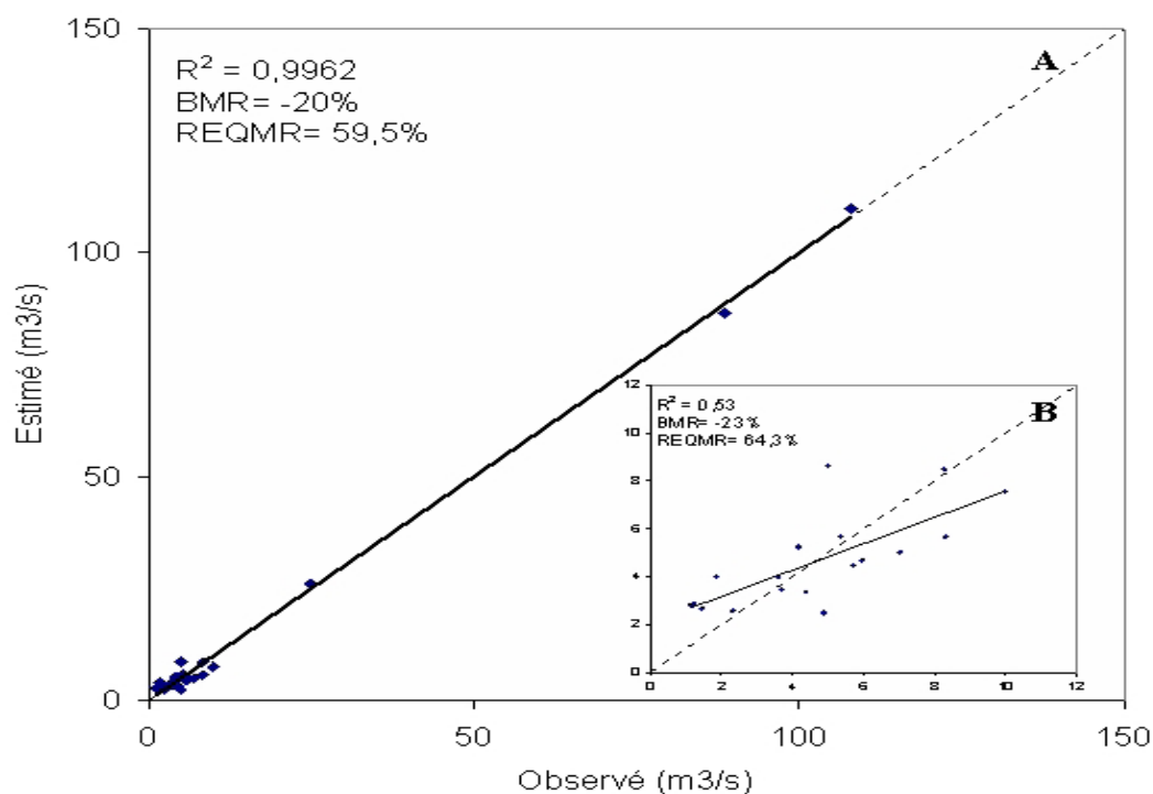
Figure 6 : Validation croisée du débit moyen interannuel estimé à l'aide de la régression simple : A) toutes les stations de jaugeage, B) excluant les trois plus grands bassins versants.
