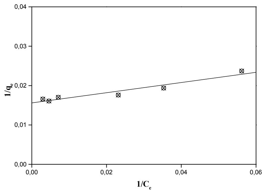
Figure 11. Application du modèle de Langmuir pour l'adsorption du rouge basique par la sciure de bois. Application of the Langmuir model to the adsorption of the basic red dye on sawdust.
