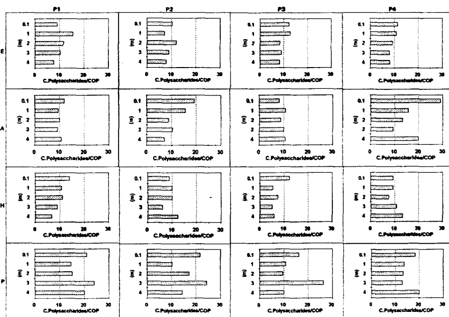
Figure 4 Évolution des teneurs en carbone des polysaccharides rapportées au COP (%) dans la colonne d'eau au cours des saisons (E, A, H et P) sur les quatre stations sélectionnées.
