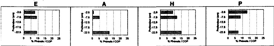
Figure 7 Évolution des teneurs en COP (%), en polysaccharides et en phénols rapportées au COP (%) dans les dépôts sélectionnés (sous table S1 et hors table S2) au cours des saisons (E, A, H et P).
