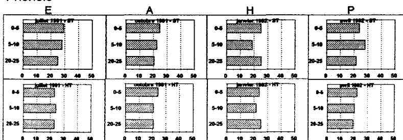
Figure 8 Pourcentages relatifs des classes majeures de composés organiques dans les dépôts sélectionnés (sous table ST et hors table HT) au cours des saisons (E, A, H et P).
