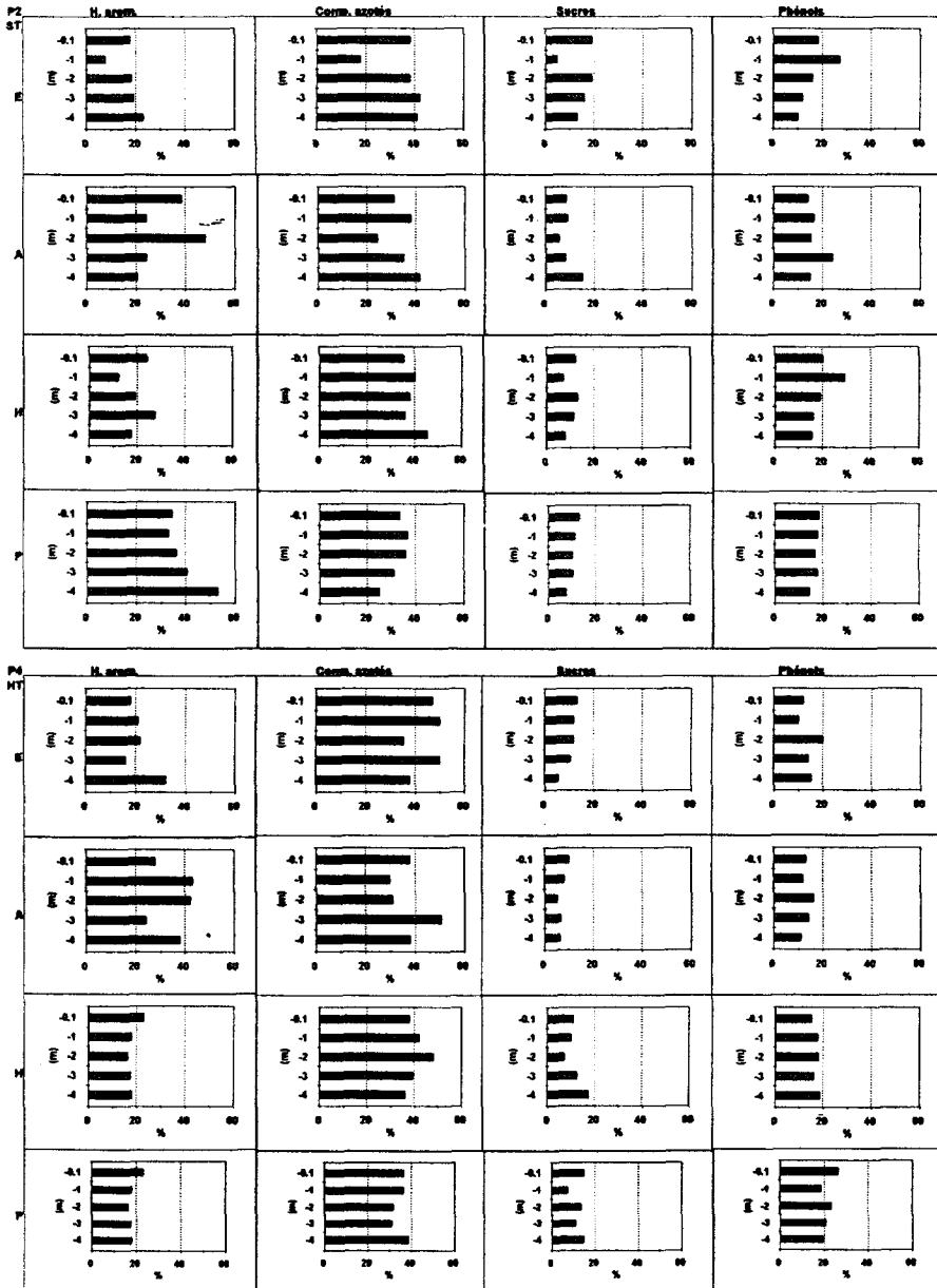
Figure 6 Pourcentages relatifs des classes majeures de composés organiques dans la colonne d'eau au cours des saisons (E, A, H et P) sur les deux stations sélectionnées sous table P2 et hors table P4 (analyse par pyrolyse).
