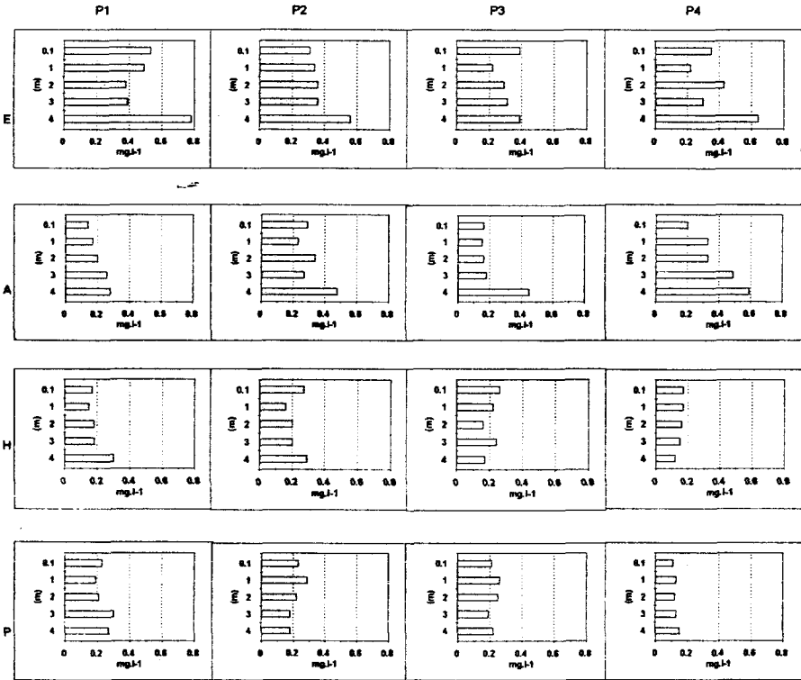
Figure 3 Évolution des teneurs en COP ( \text{mg}\cdot\text{l}^{-1} ) dans la colonne d'eau au cours des saisons (E, A, H et P) sur les quatre stations sélectionnées.
