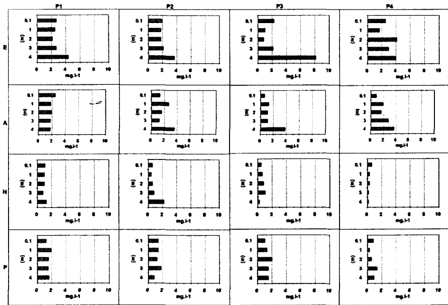
Figure 2 Évolution de la charge en suspension ( \text{mg}\cdot\text{l}^{-1} ) dans la colonne d'eau au cours des saisons (E, A, H et P) sur les quatre stations sélectionnées.
