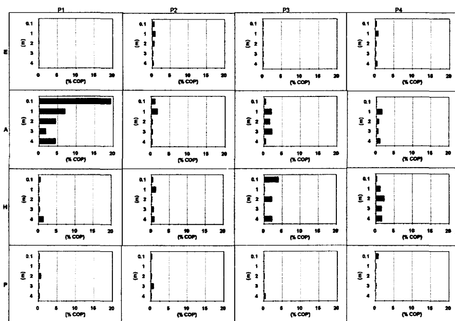
Figure 5 Évolution des teneurs en composés phénoliques rapportées au COP (%) dans la colonne d'eau au cours des saisons (E, A, H et P) sur les quatre stations sélectionnées (analyse CLHP).
